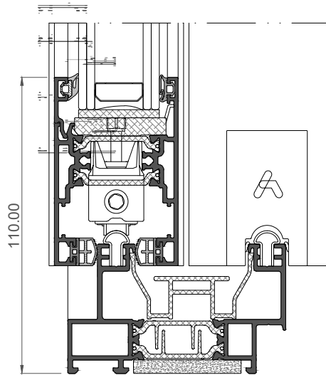
Sección 2 / Section 2
