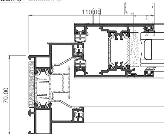
Sección 3 / Section 3
