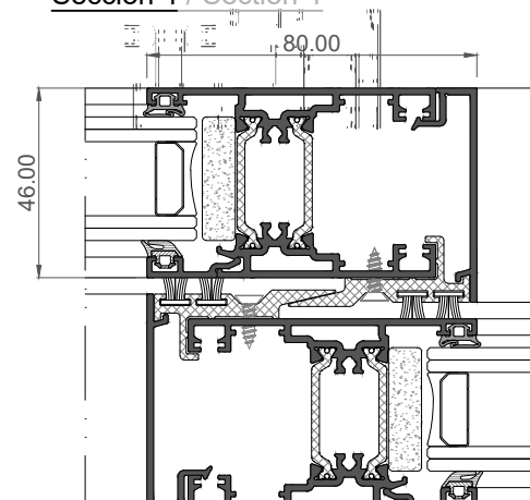
Sección 4 / Section 4
