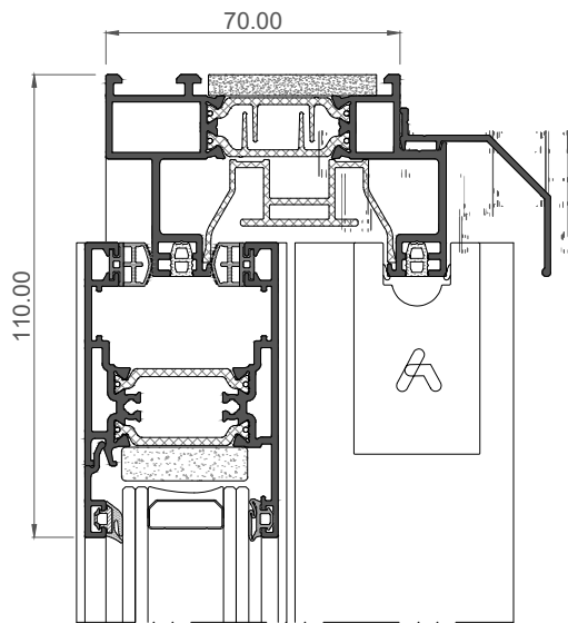
Sección 1 / Section 1
